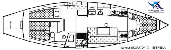
Layout SKORPION II ESTRELLA
